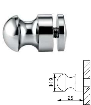
Item No : DK13 Back-to Back Knob
