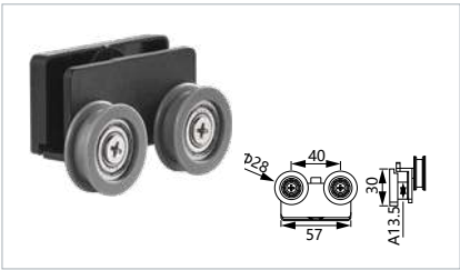
Item No: SDR70 Shower door roller Materail:SUS304
