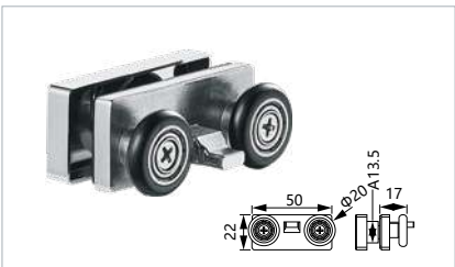
Item No: SDR69 Shower door roller Material:SUS304
