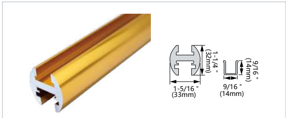
Item No: MW04 Header Support Bar
