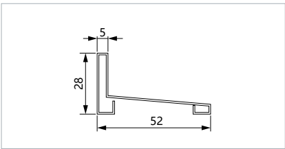
③ MD2-C ▪ Bottom Sill
