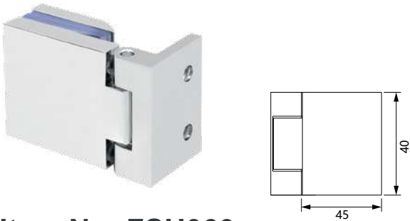
Item No: FSH060 Wall Mount Hinge
